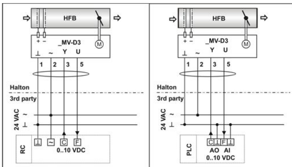
1C System med rumstermostat 1D Styrssystem för byggnaden
