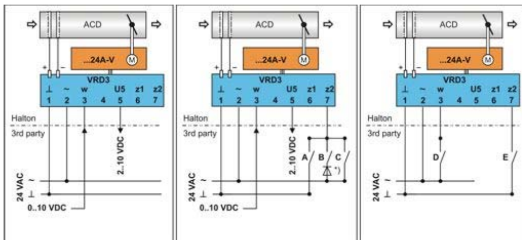
2 A. Normal styrning 2B Dominerande styrning 2 C. Styrning med konstant luftflöde
