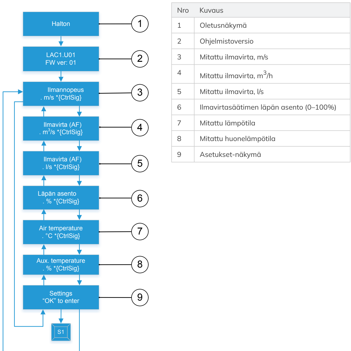
Kuva 15. Halton Max Ultra Circular (MUC) -ilmavirtasäätimen aloitusnäköymät
