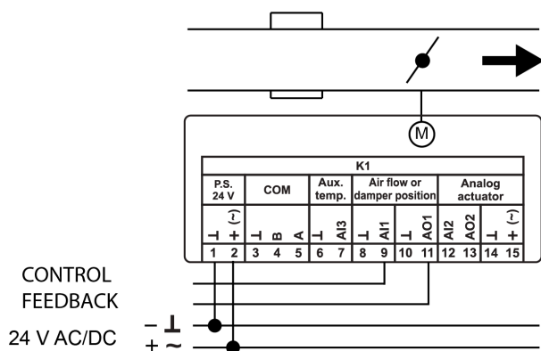
Kuva 17. KytKentäkaavio Analoginen säätö
