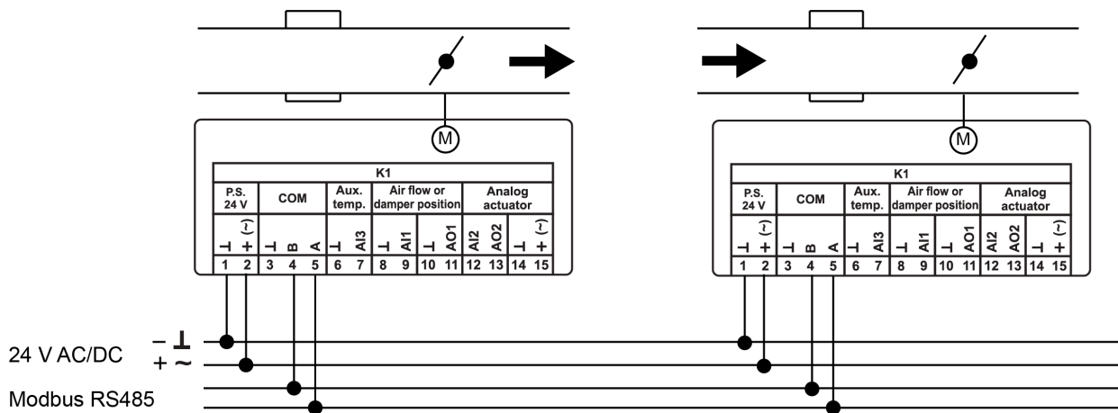
Kuva 18. Kytkentäkaavio Modbus-tiedonsiirto
