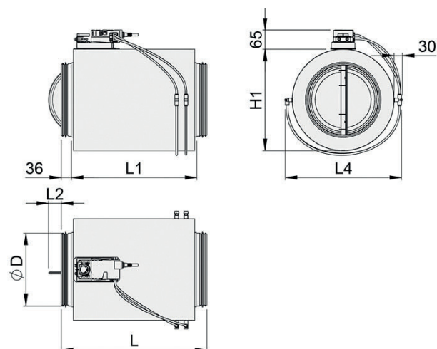
Halton Max MLC/I, modèle avec isolation (50 mm)
