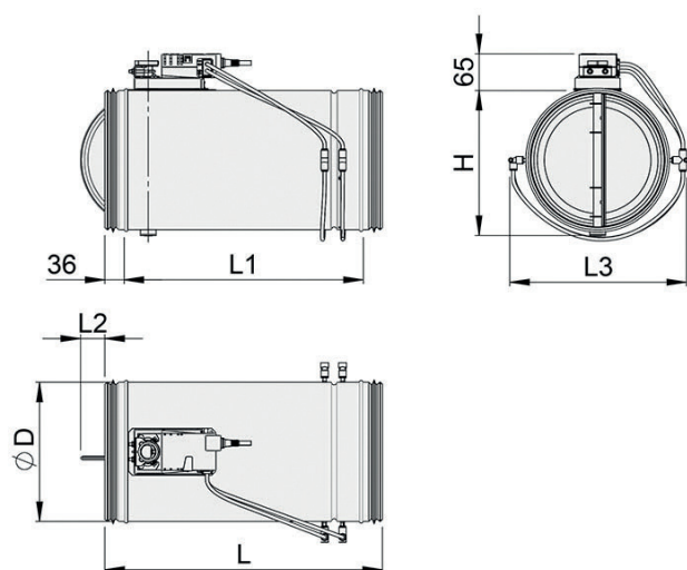
Halton Max MLC/G, modèle sans isolation
