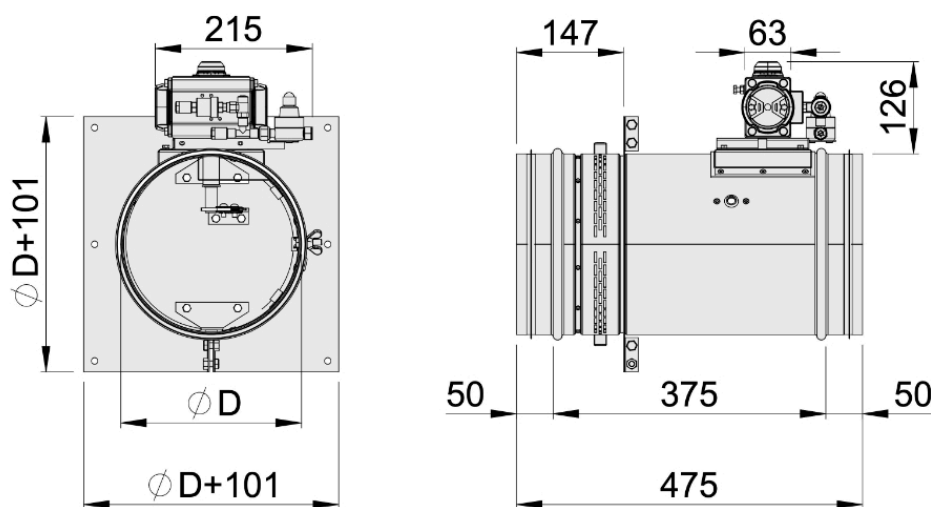
Fig. 2. Halton Ivo ITC dimensions
