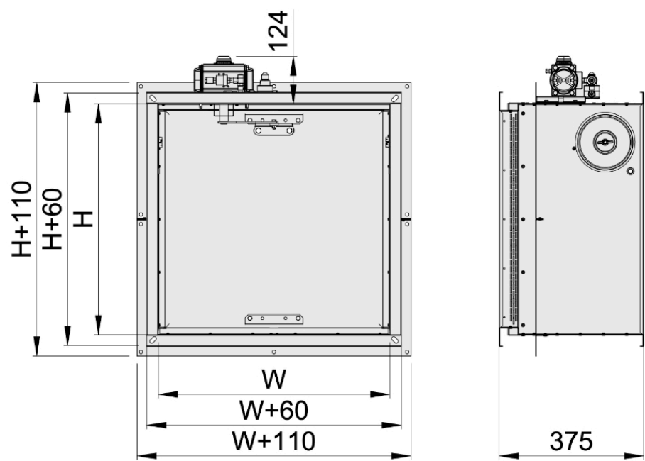
Fig. 2. Halton Ivo ITR dimensions
