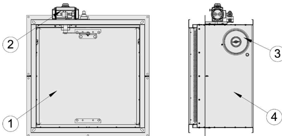
Fig. 1. Halton Ivo ITR structure
