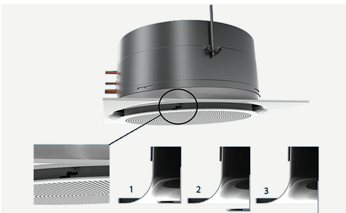
Pos. 1 = encastrée Pos. 2 = réhaussée Pos. 3 = Boost
