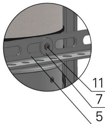
Kuva 16 Ripustusrenkas ja asennuskisko yhdistetty ruuvilla tai niitillä
