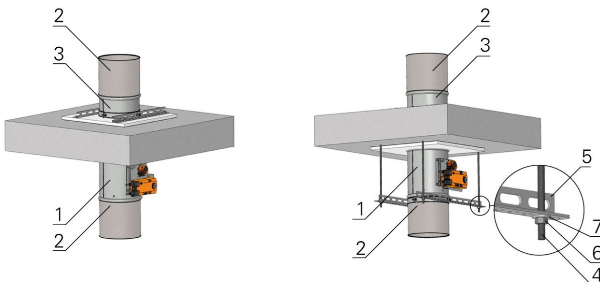
Kuva 14 Toimintamekanismi lattiarakenteen alapuolella
