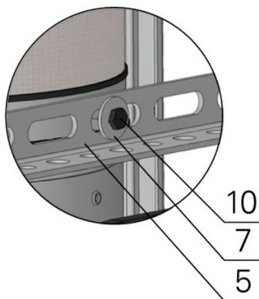
Kuva 15 Ripustusrenkas ja asennuskisko yhdistetty pultilla
