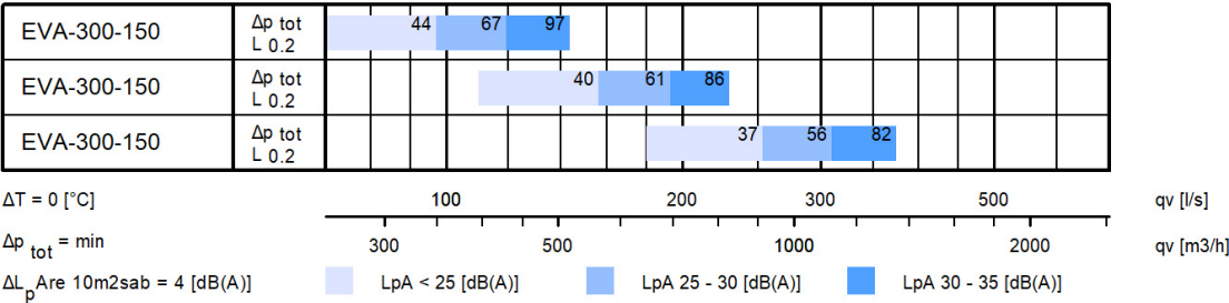
Fig.1. Without plenum
