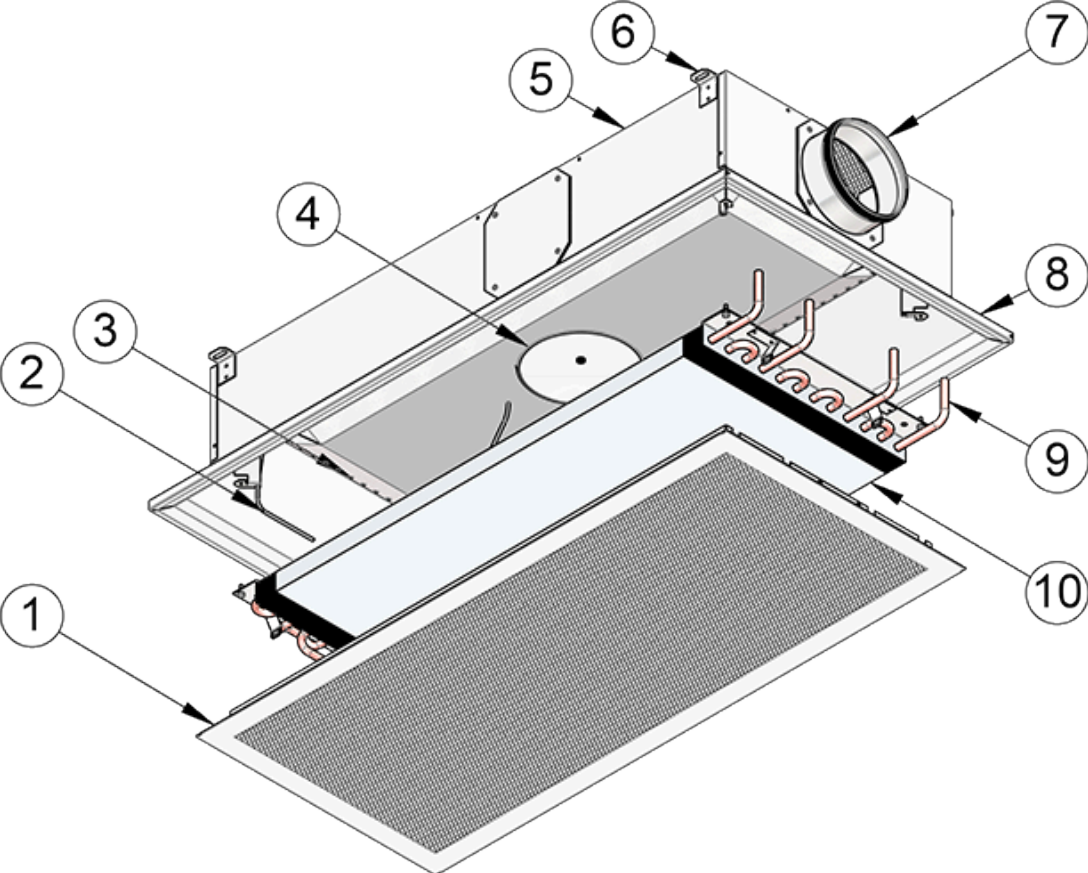
Fig.20. Halton Rex RXP
