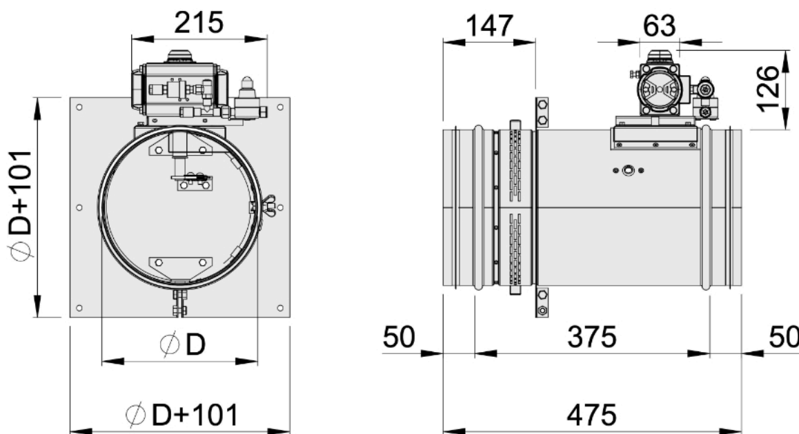
Fig. 2. Halton Ivo ITC dimensions
